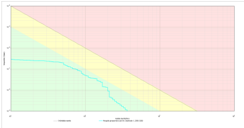
Abbeelding 3: fN-curve plangebied in de beoogde situatie (huidige vervoerscijfers)
